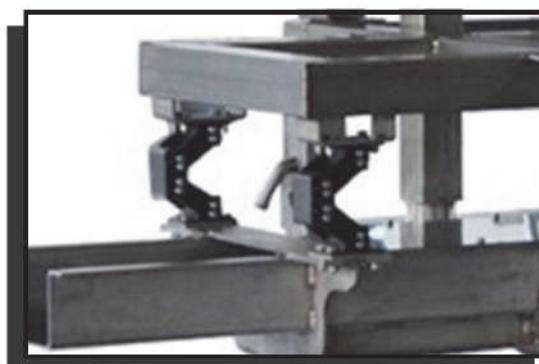
VIB DE-2L в вибрационной машине
