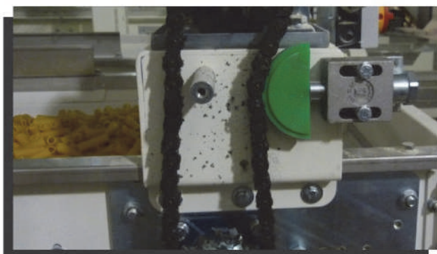
Натяжитель TEN BLOC в конвейере для макаронных изделий
