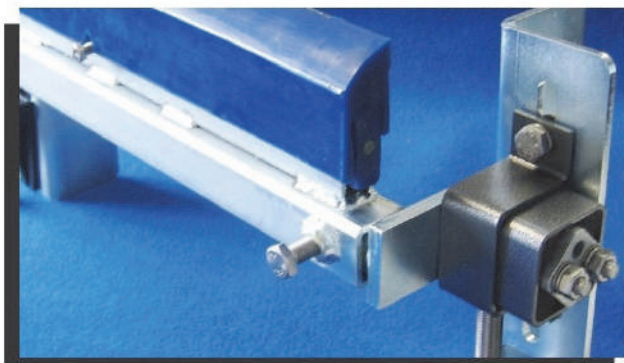
VIB AR-P используется как опора для ленточного скребка
