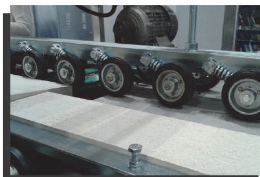
Натяжитель ARCO в отрезной машине
