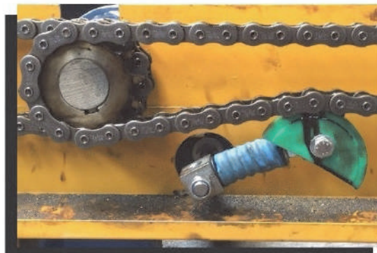
Натяжитель ARCO в конвейере
