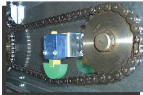
Натяжитель BLU в сборщике яиц
