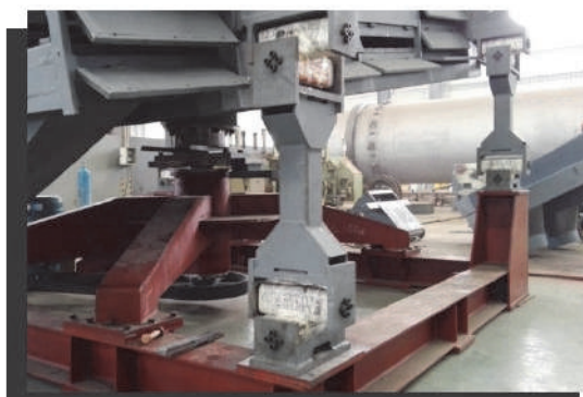
VIB CR-P в инерционном грохоте
