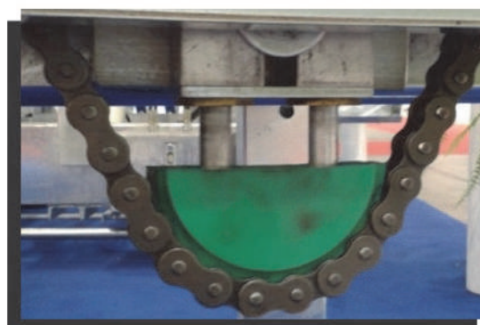
Натяжитель ASSO в упаковочной машине
