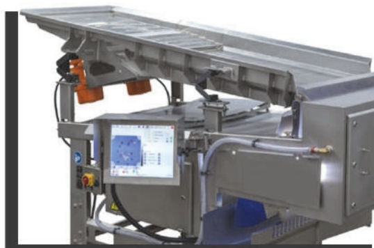
Нержавеющая вибрационная опора VIB DE 40R
