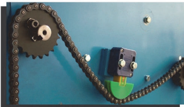
Натяжитель BLU в птицефабрике
