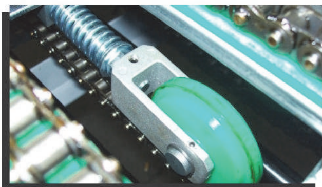
Натяжитель ARCO в упаковочной машине
