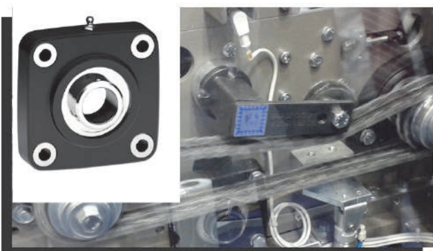
Подшипниковый узел из пластика UCF и натяжитель CRESA RE
