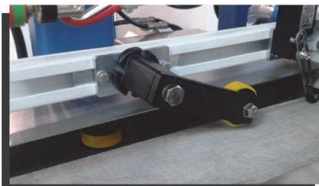
СIAO PX-R в станке для снятия фаски
