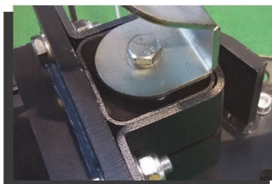
VIB AR-T в подметательной машине
