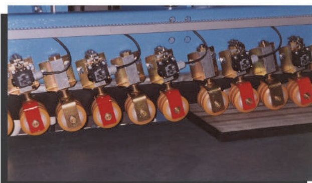
Натяжители ASSO в кромкооблицовочных станках
