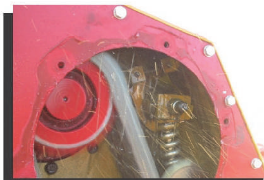
Натяжитель ARCO в сельхоз мульчере
