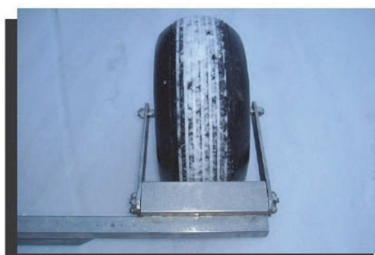
VIB AR-P в Кайт-багги
