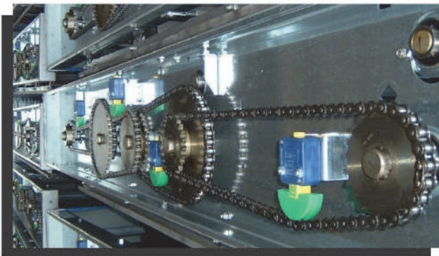
Сборщик яиц
